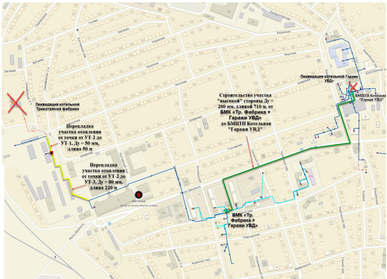
Рисунок 12 – Строительство и реконструкция участков сети для объединения систем теплоснабжения котельных «Гаражи УВД», «Орентрикотаж»
