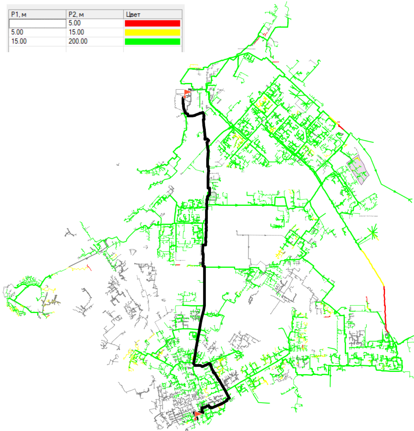
Рисунок 1 – Графическая интерпретация с располагаемыми напорами системы теплоснабжения Сакмарской ТЭЦ к 2044 году, БЕЗ увеличения диаметров квартальных трубопроводов.
