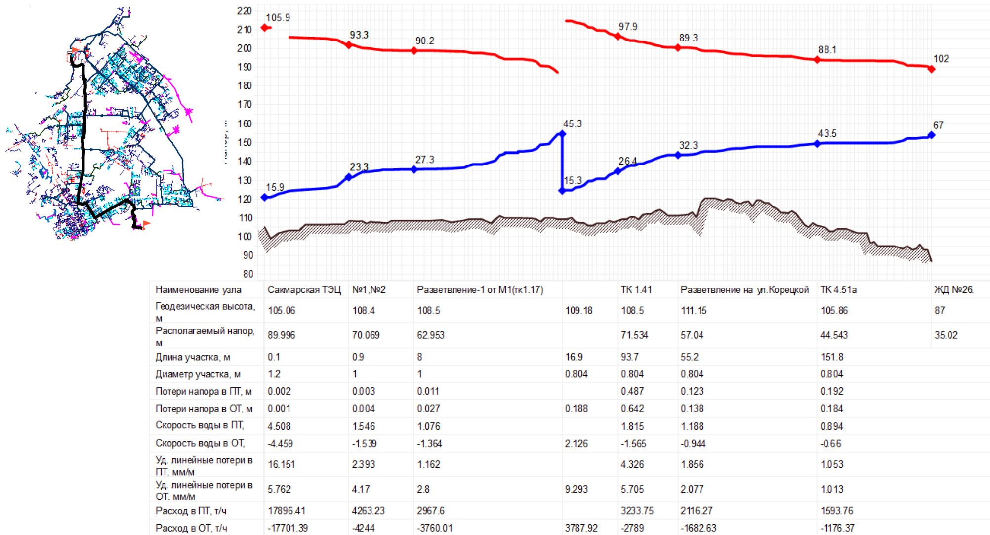
Рисунок 3 – Пьезометрический путь от Сакмарской ТЭЦ до наиболее отдалённого потребителя ЖК «Дубки» (16 км). Располагаемый напор 35 м вод. ст. Потребитель подключен по независимой схеме.
