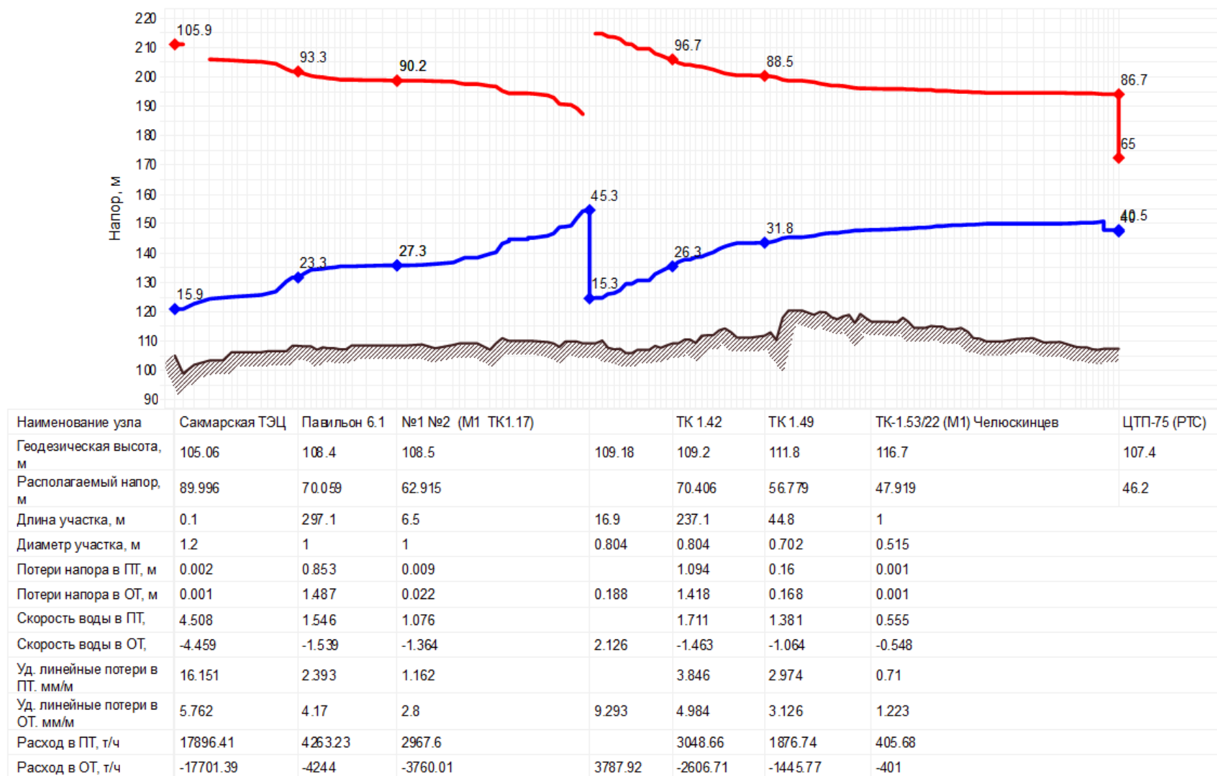
Рисунок 2 – Пьезометрический путь от Сакмарской ТЭЦ до наиболее отдалённого потребителя ЦТП №75 (17 км). Располагаемый напор 46 м вод. ст. Потребитель подключен по независимой схеме.
