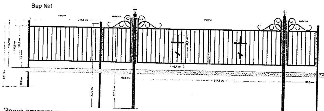
Эскиз ограждения
