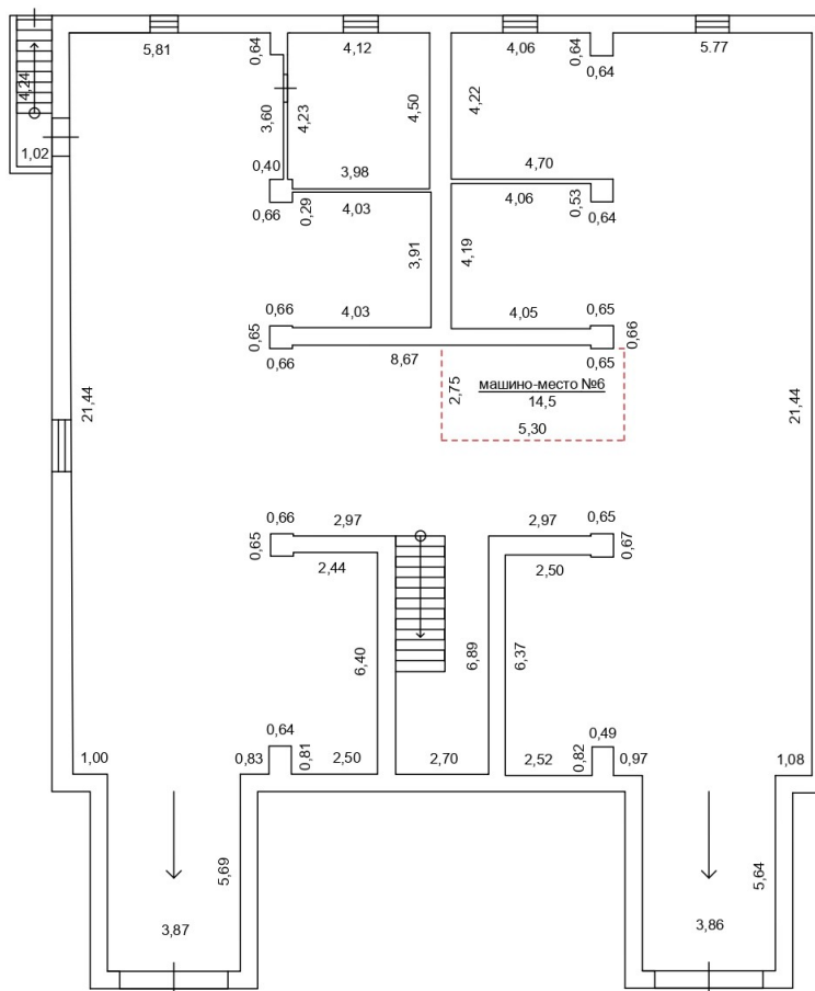
Фрагмент графической части проекта технического плана образуемого машино-места (цокольный этаж)
