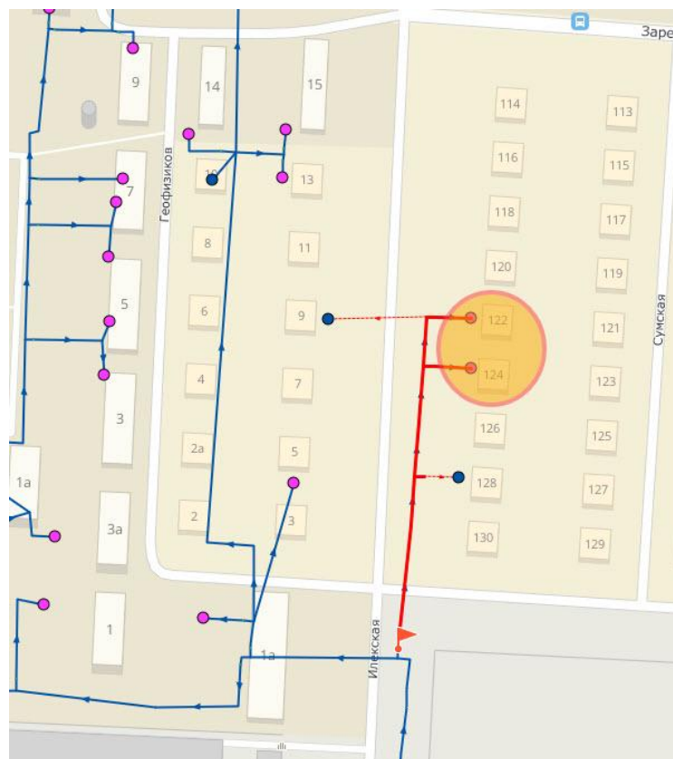
Рисунок 1 – Схема трубопроводов до домов ул. Илекская д. 122, д. 124
